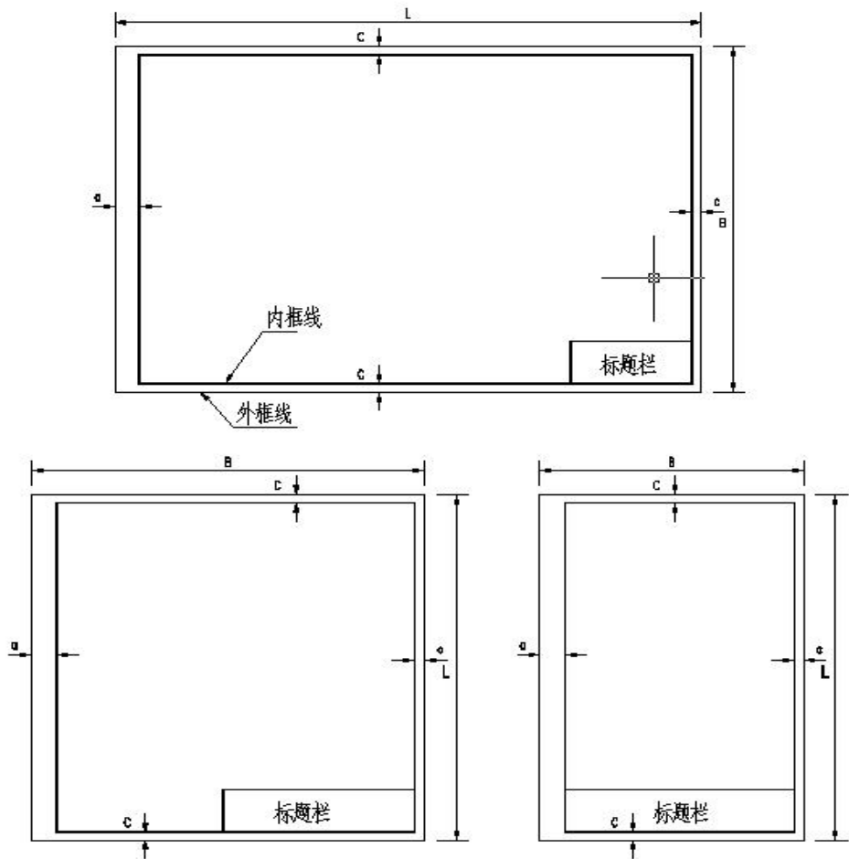
图 1： 图框
